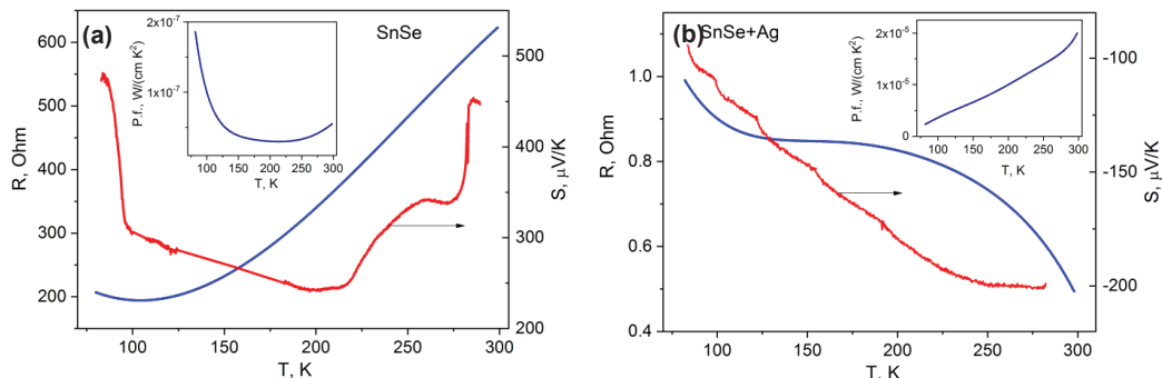
Рис. 2. Температурные зависимости сопротивления R и термоэдс S слоев SnSe. На вставке представлена температурная зависимость фактора мощности Pf=S^2\sigma . (a) – нелегированный образец SnSe; (b) – легированный Ag образец SnSe
