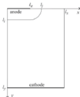
Fig. 1. Geometria diodei semiconductoare
