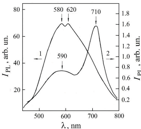
Рис.2. Спектры фотолюминесценции монокристаллов CdSe, выращенных по методу Бриджмена. T = 300K. Кривые: 1 – исходный, неотожженный кристалл, 2 – кристалл, отожженный в расплаве Cd
