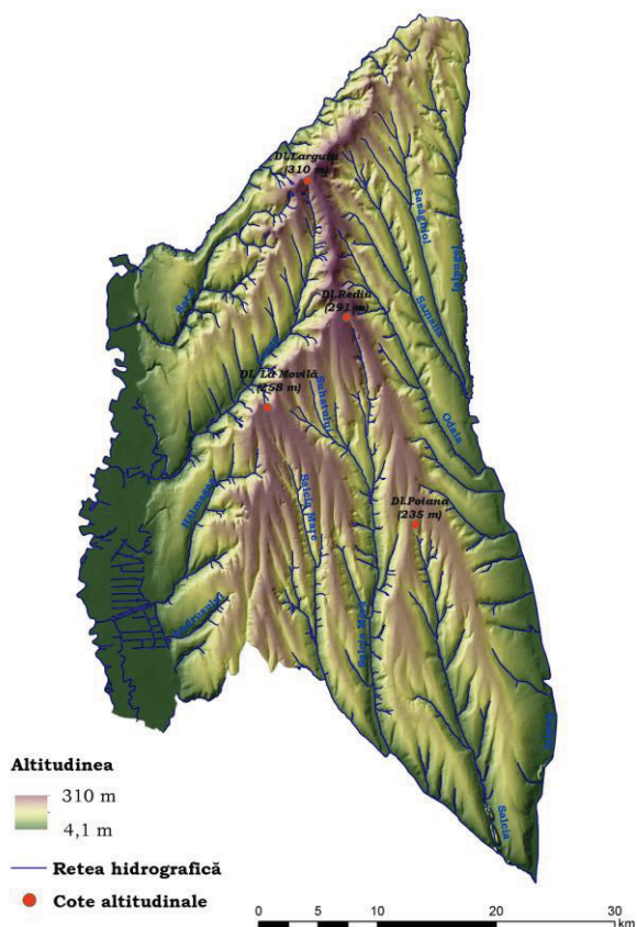
Fig. 1. Rețeaua hidrografică din Colinele Tigheciului
