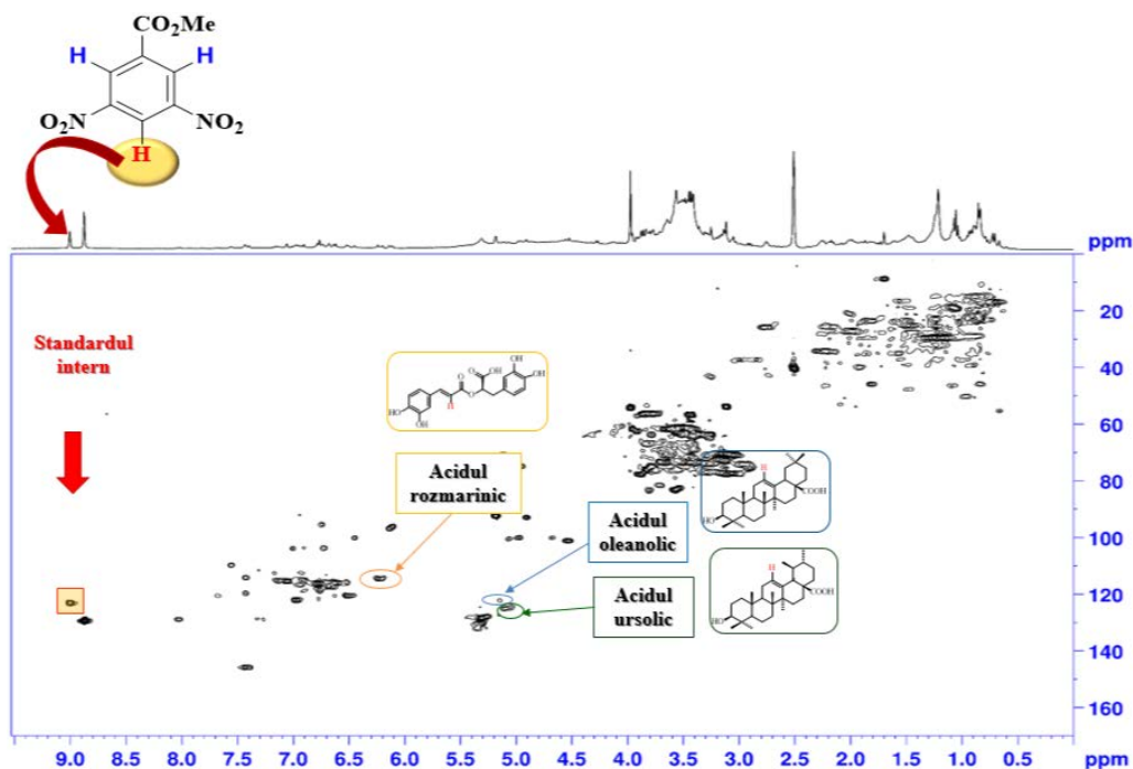
Figura 3. Spectrul RMN pentru o mostră reprezentativă de extract de mentă
