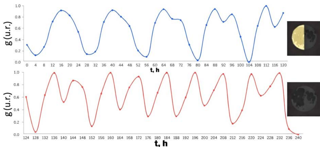
Fig.1. Variația accelerației căderii libere timp de 10 zile
