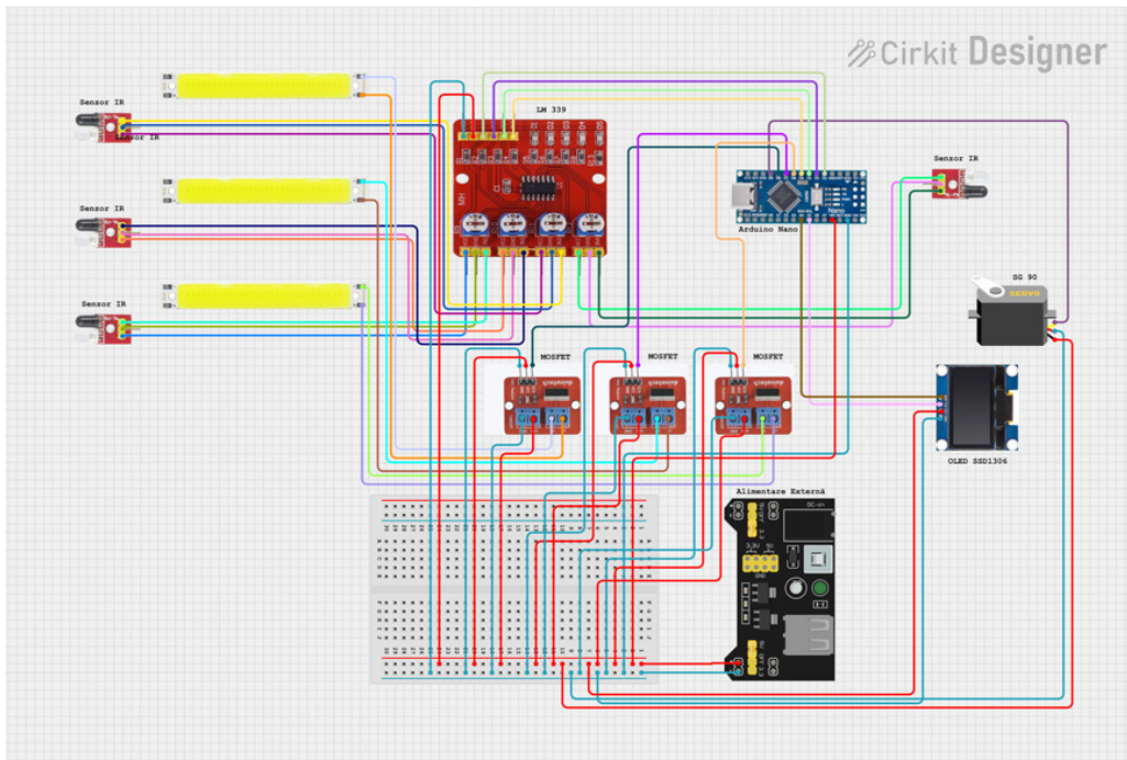
Fig.1. Schema de interconectare a modulelor
