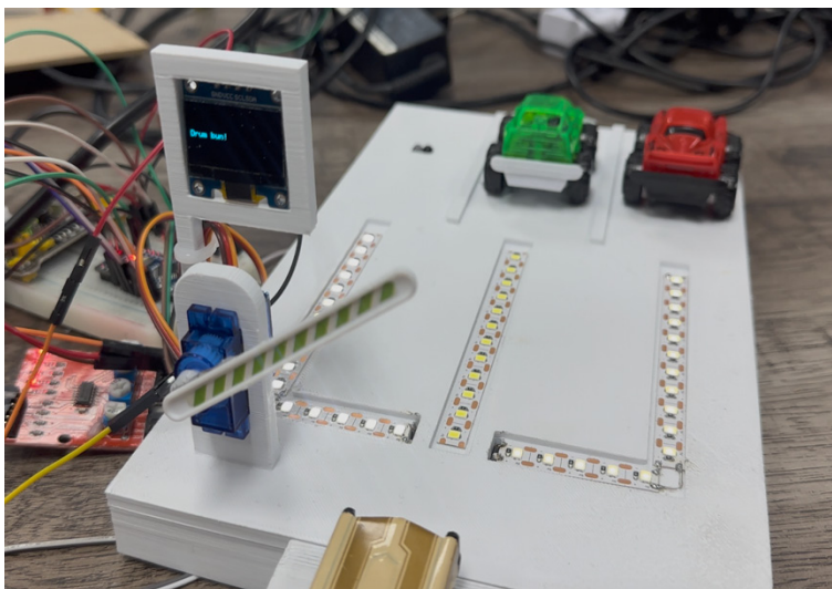
Fig.2. Rezultatul testului: Loc liber identificat, afișaj actualizat, barieră deschisă și banda LED activată
