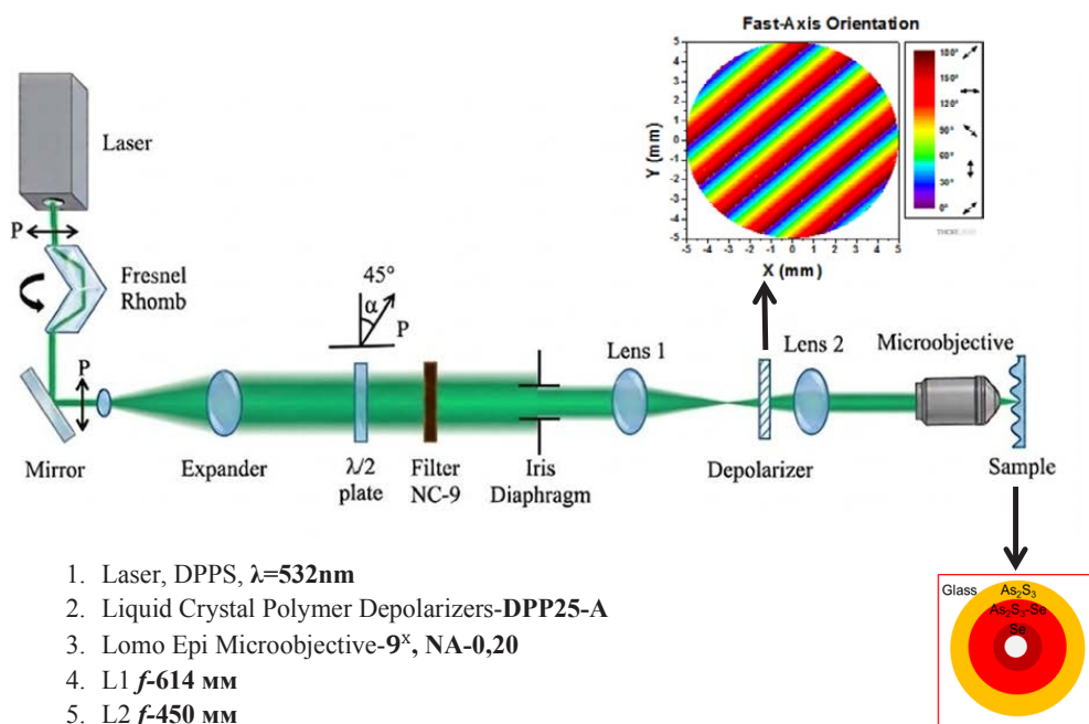
Рисунок 1. Схема экспериментальной установки для формирования поверхностных решеток методом пространственно-неоднородной поляризации
