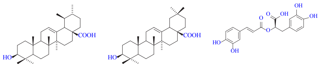
Figura 2. Acidul ursolic (1), acidul oleanolic (2) și acidul rozmarinic (3)
