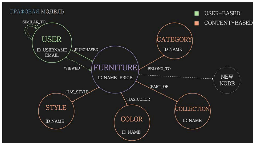
Рисунок 2. Графовая модель
