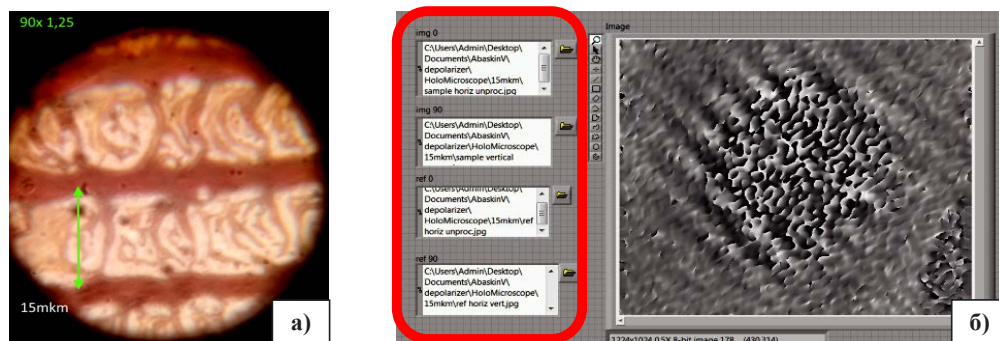
Рисунок 2. Изображение решетки в светлом поле и на голографическом микроскопе. Красный овал - 4 поляризационных голограммы \perp и \parallel .
