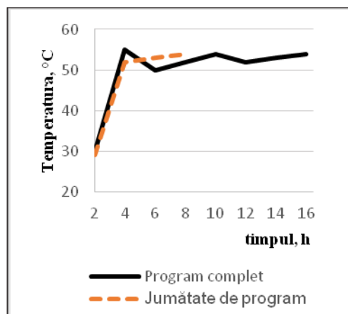
Figura 4. Variația temperaturii în interiorul sterilizatorului încărcat în funcție de timp. Condiții: [EtO] = 882 mg·h/L; Rh = 56%
