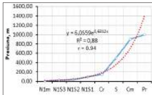
Figura 2. Dependenta presiune hidrostatică-acvifer apa – acvifer (albastru-reală, roșie – statistică)
