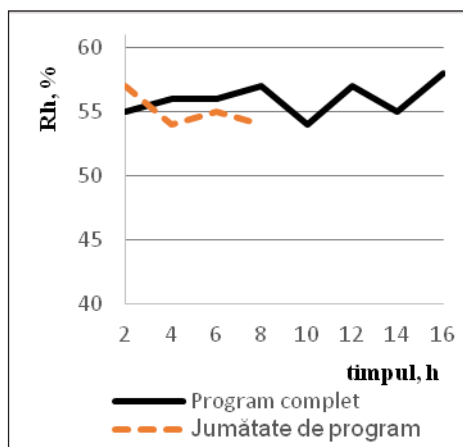
Figura 5. Variația umidității în interiorul sterilizatorului încărcat în funcție de timp. Condiții: [EtO] = 882 mg·h/L; t = 53°C
