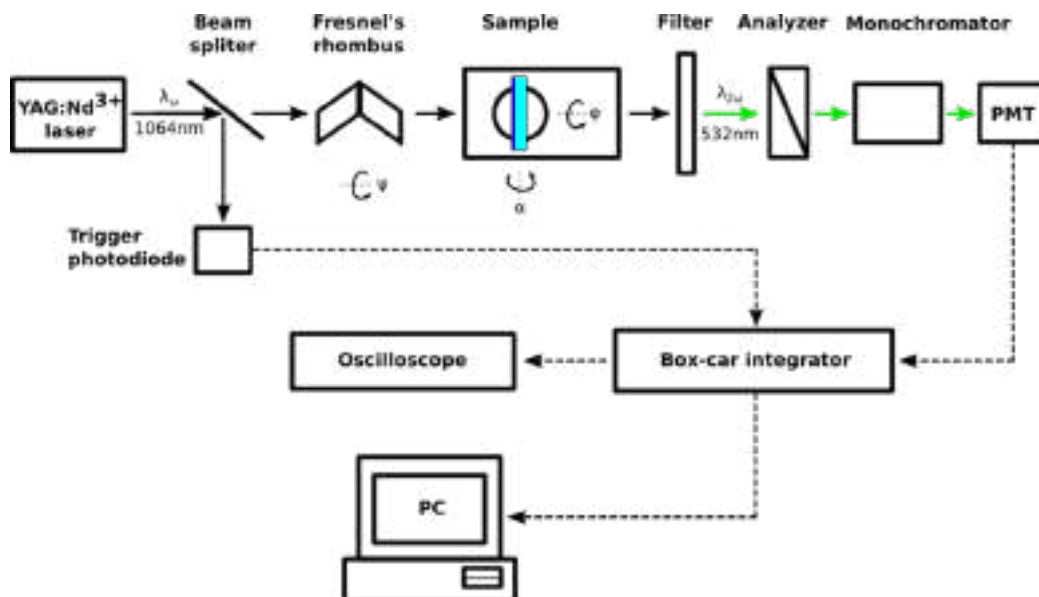
Figura 1. Schema configurației experimentale pentru măsurători ale armonicei secunde optice în transmisie
