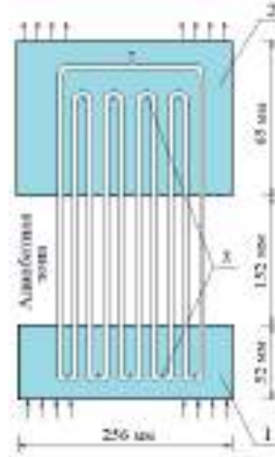
Рисунок 3. Схема ПТТ: 1 – зона испарения; 2 – зона конденсации; 3 – термопары
