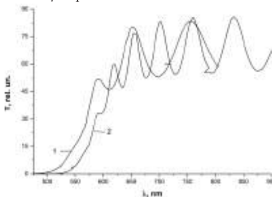
Figura 5. Spectrele de transmisie ale peliculei subțiri amorfe \text{As}_{45}\text{S}_{15}\text{Se}_{40} inițial (1) și după expunerea cu lumină ultravioletă (2)
