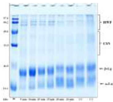
Figura 3. SDS-PAGE 15% a proteinelor solubile extrase soluția tampon, pH 8.0, din CPM, obținute la electroactivarea ZCÎP, în EDC-3, regim periodic, j=20\text{mA}/\text{cm}^2 (M – marker, 5-20 min – durata de procesare, 15 min sp, 20 min sp, CC sp, obținute din \text{CPM}_2 CC – conținutul celulei catodului)
