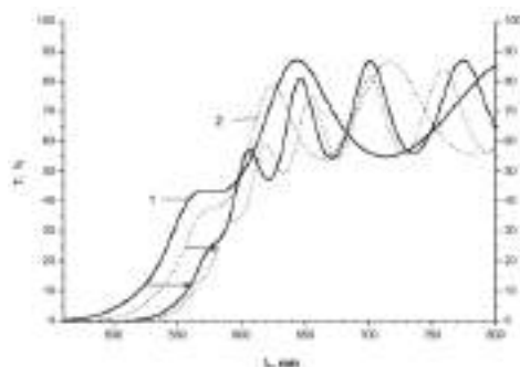
Figura 6. Spectrele de transmisie ale peliculelor subțiri amorphe (As_{45}S_{15}Se_{40})_{1-x}Sn_x cu (x=0 (1) și 0.1 (2) inițial și după expunerea cu lumina ultravioletă
