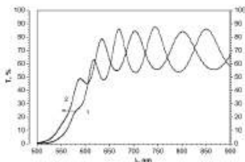
Figura 7. Spectrele de transmisie ale peliculelor subțiri amorphe As_{45}S_{15}Se_{40} , după expunerea luminii violette inițial (1) și ulterior după tratarea termică (2)
