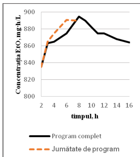
Figura 6. Variația concentrației EtO în interiorul sterilizatorului încărcat în funcție de timp. Condiții: t = 54°C; Rh = 56%
