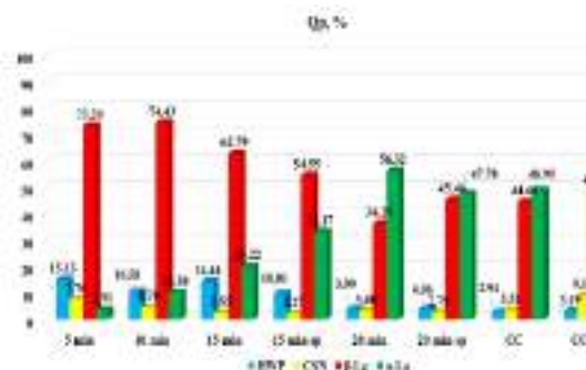
Figura 4. Variația procentuală Q_p , % a recuperării fracțiilor proteice în CPM, obținute la electroactivarea ZCÎP în EDC-3, regim periodic, j=20\text{mA}/\text{cm}^2 (5-20 min – durata de procesare, 15 min sp, 20 min sp, CC sp, obținute din \text{CPM}_2 CC – conținutul celulei catodului)
