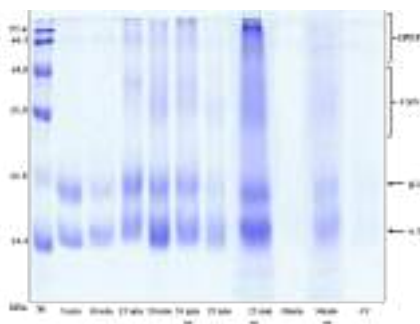
Figura 6. SDS-PAGE 15% a proteinelor solu- bile extrase soluția tampon, pH 8.0, din CPM, obținute la electroactivarea ZCSP, în EDC-pi- lot, regim periodic, j=10\text{mA/cm}^2 (M – mar- cher, 5-30 min – durata de procesare, 20 min sp, 25 min sp, 30 min sp obținute din CPM 2 , CC – conținutul celulei catodului)
