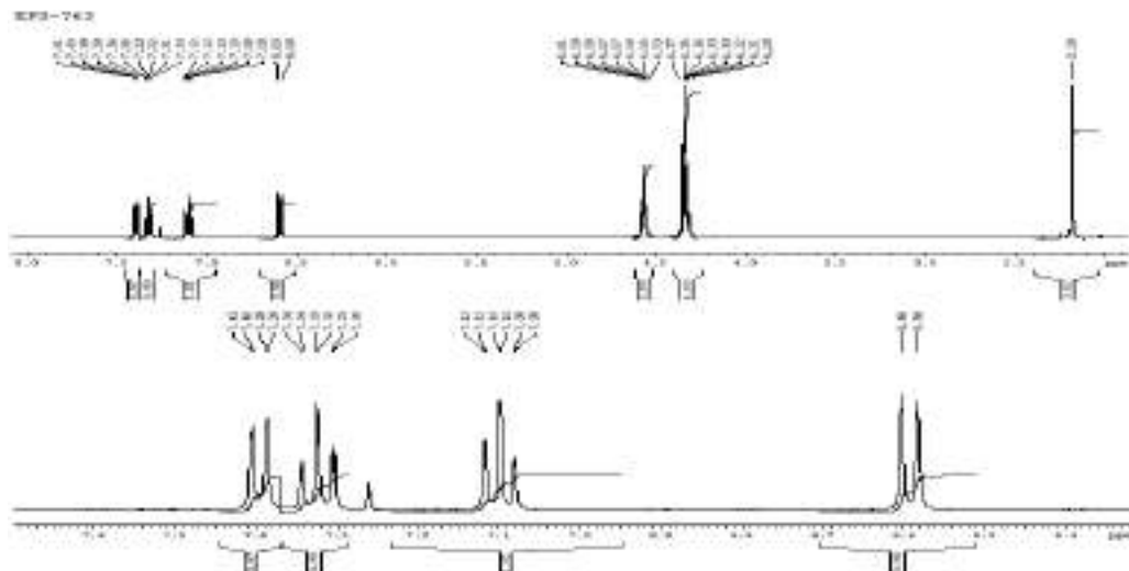
Figura 2. Spectrul ^1\text{H} RMN al compusului 4
