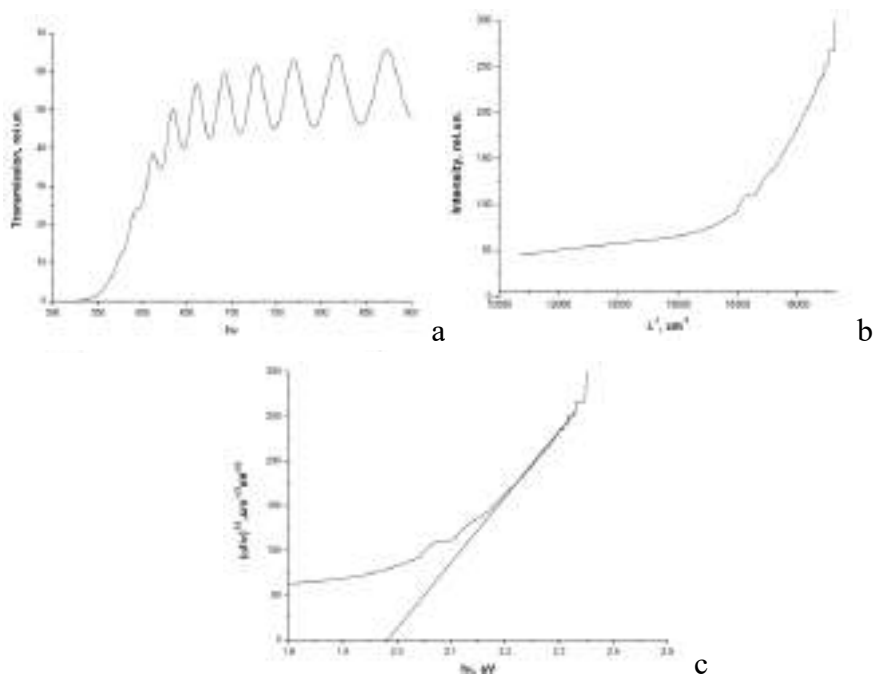
Figura 4. Spectrele de transmisie a peliculei subțiri amorfe \text{As}_{45}\text{S}_{15}\text{Se}_{40} ( x=0 ) (a), de absorbție (b) și dependența spectrală în coordonatele lui Tauc ( E_g \equiv 1.98 \text{ eV} ), (c). Grosimea probei d=1982 \text{ nm}
