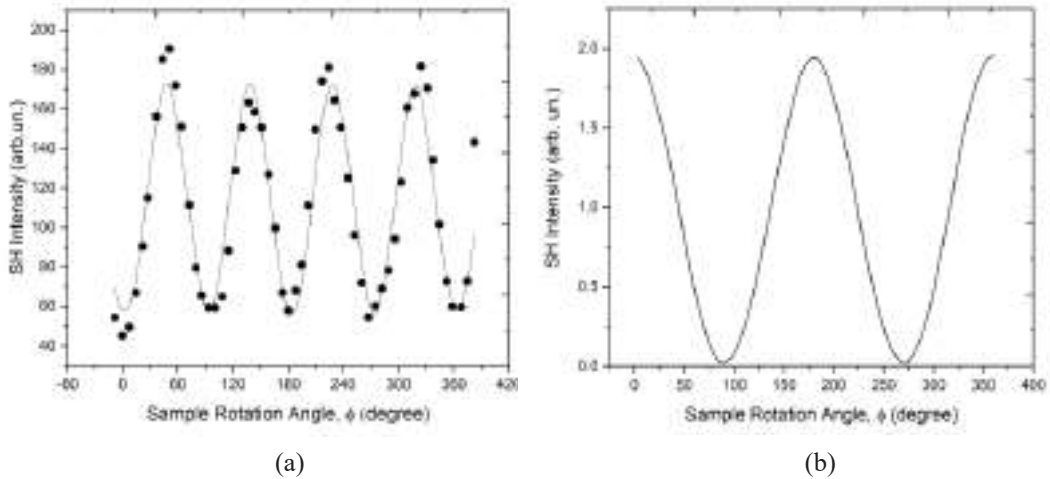
Figura 4. (a) Intensitatea semnalului AS s-polarizat generat de fasciculul fundamental s-polarizat în funcție de unghiul de rotație \varphi al eșantionului I_{ss}^{SH}(\varphi) : cercurile – datele experimentale; linia continuă reprezintă rezultatul calculului în baza ecuației (5).
